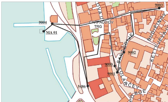
Nivelmanska mreža mareografske postaje Koper (vir: DPK-1000 GURS)
